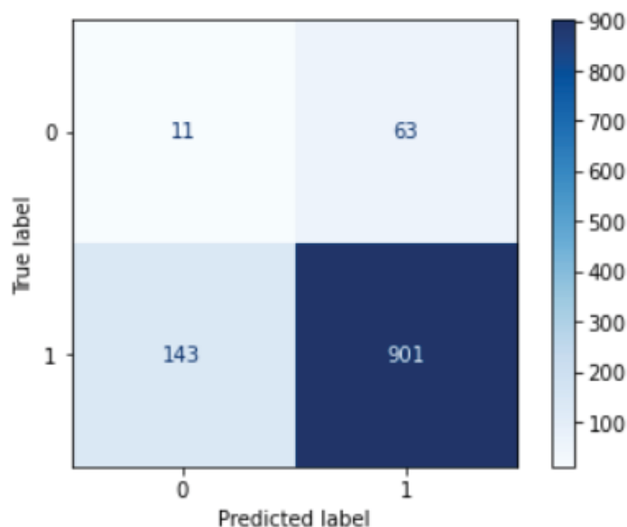
Figure 2. Matrice de confusion du modèle de régression logistique
