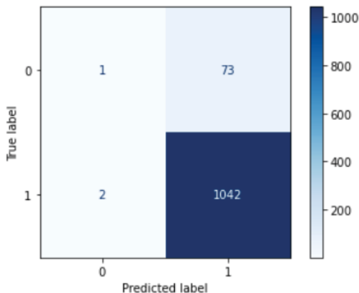
Figure 3. Matrice de confusion de l'arbre de décision
