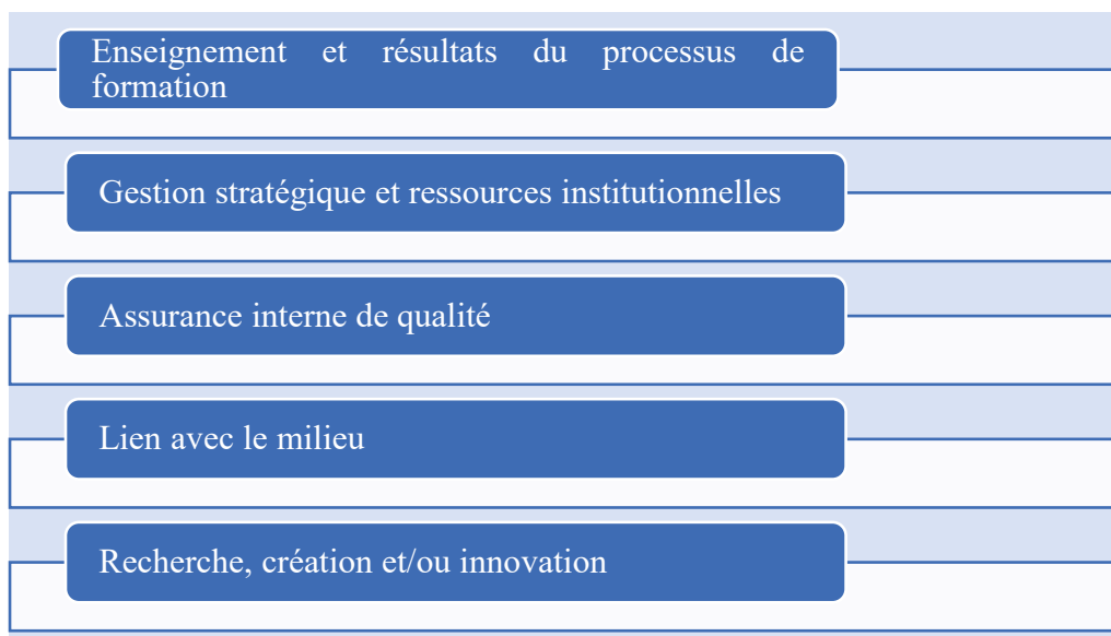
Figure 1. Dimensions évaluatives d'accréditation institutionnelle
