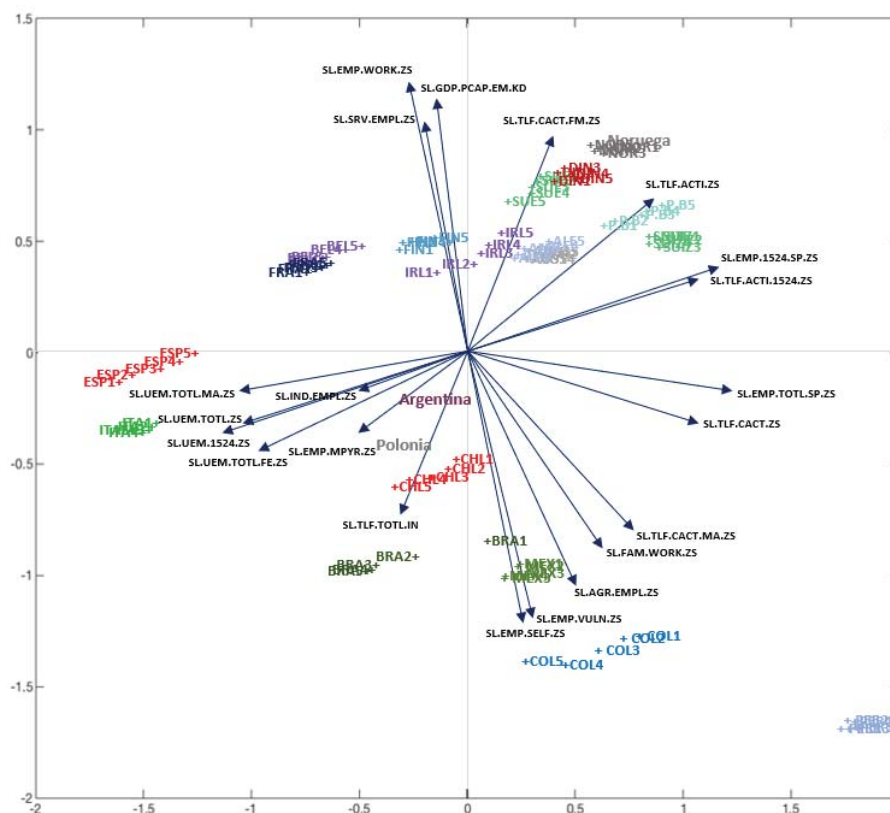
Figure 1. Représentation Consenso dans le plan 1-2
