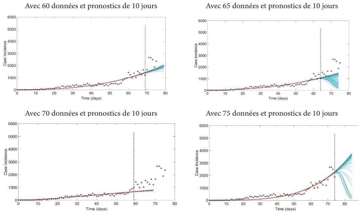
Figure 2. Modèle de Richards et sa progression
