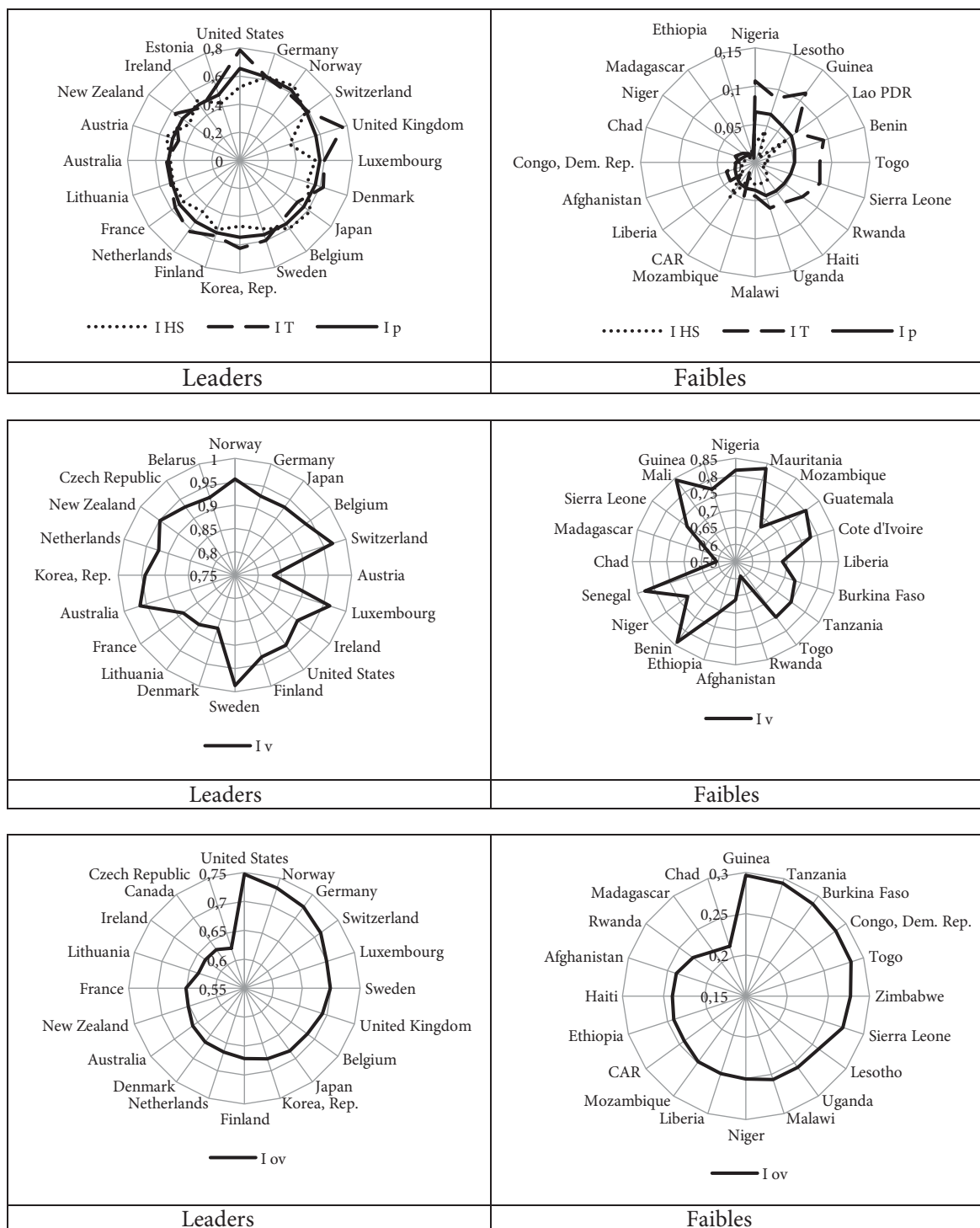
Figure 1. Index global et ses sous-index
